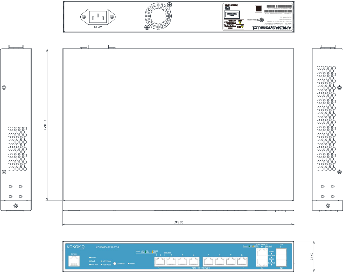
図 10-1 KOKOMO-S212GT-P 外観図
