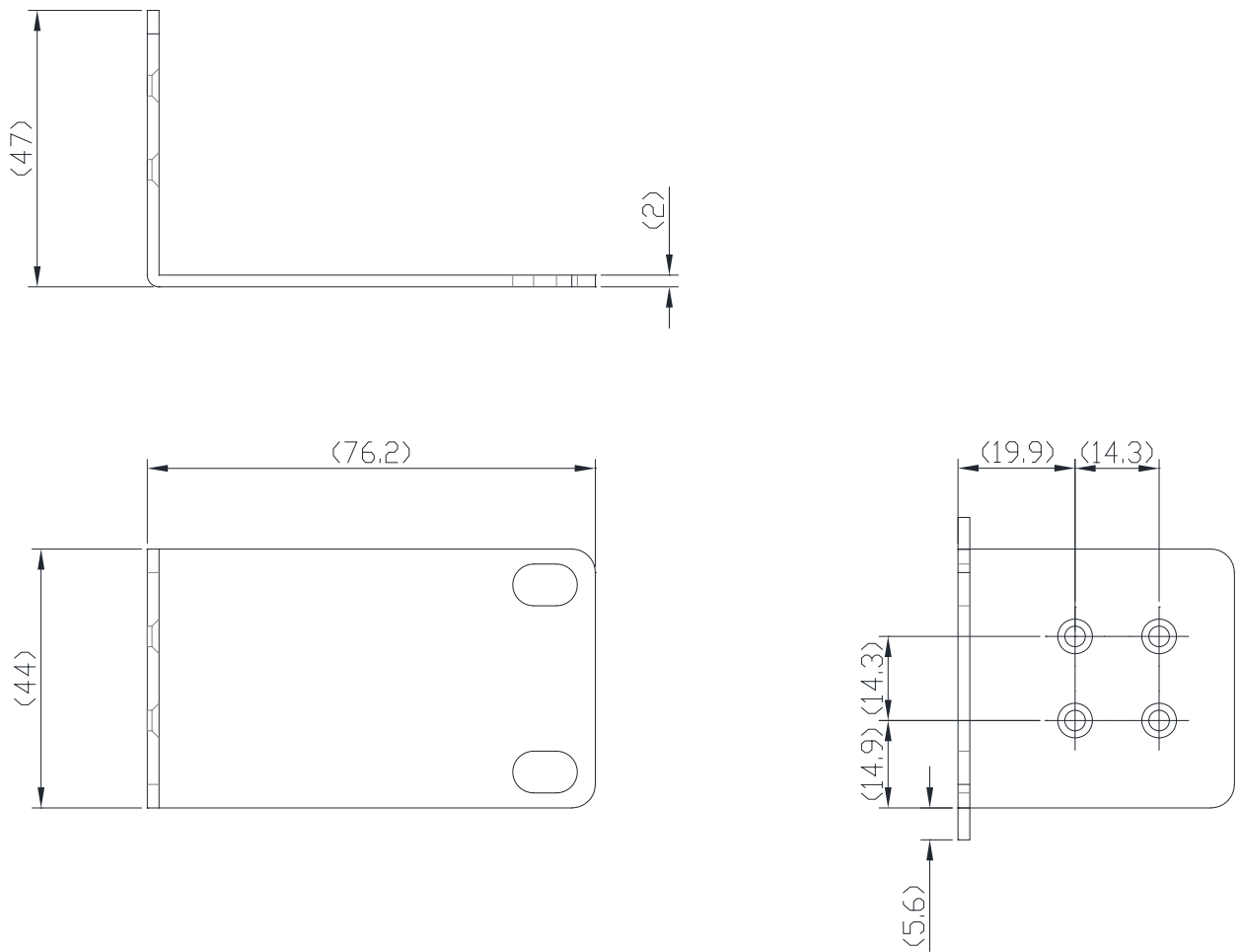
図 10-2 ラックマウント金具外観図
