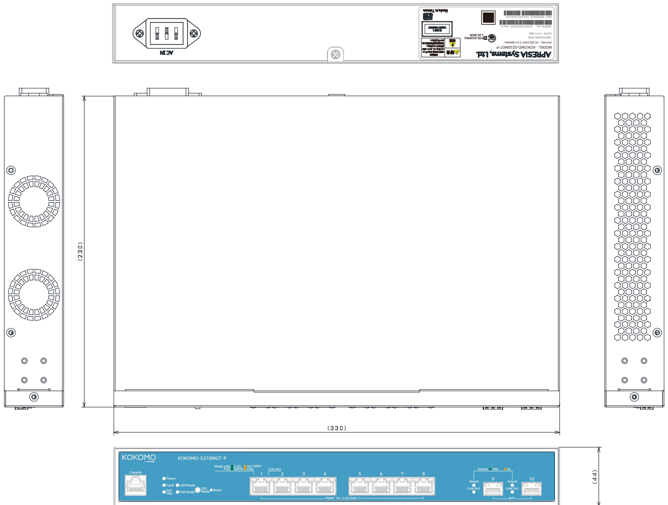
図 10-1 KOKOMO-S210MGT-P 外観図
