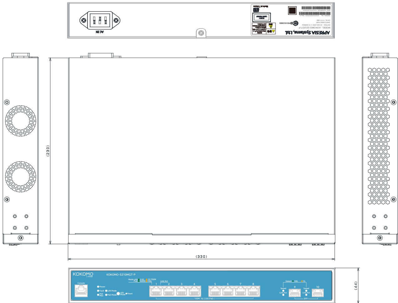
図 10-1 KOKOMO-S210MGT-P 外観図
